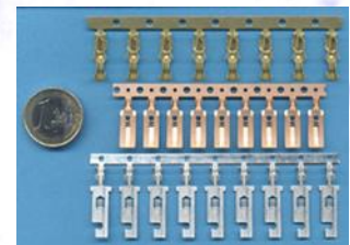
Stanzen, galvanisieren
